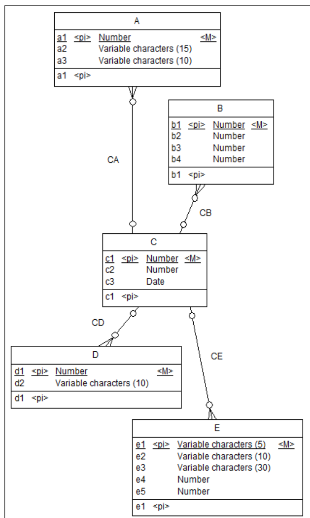
Figura 11 - DER
